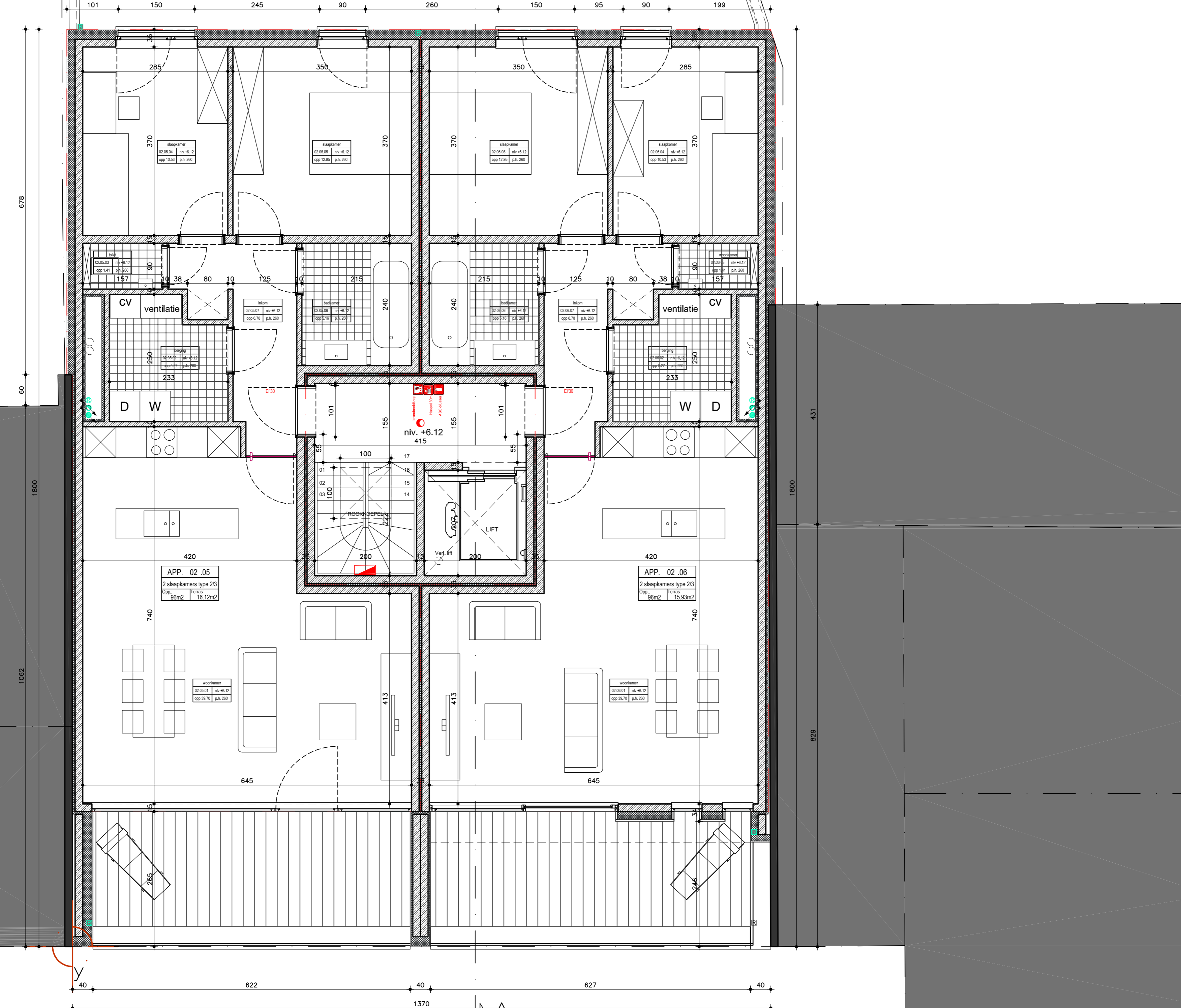
PLAN VERDIEPING +2
